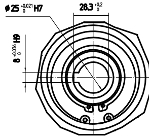
Dettaglio A scala 1:1 Rapporto 1:24 e 1:38.3
